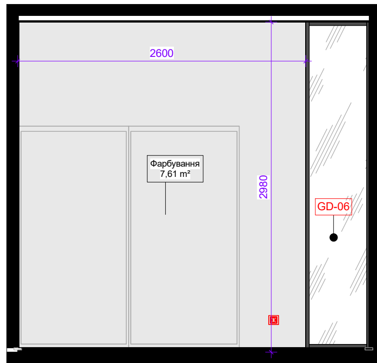
WG-02 1 : 35
