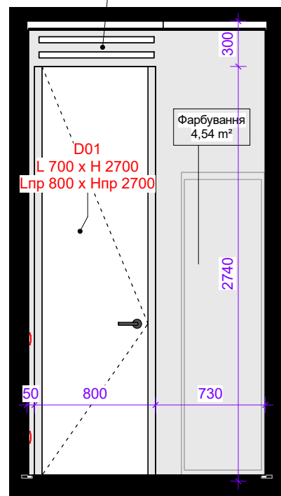
WG-01 1 : 35
