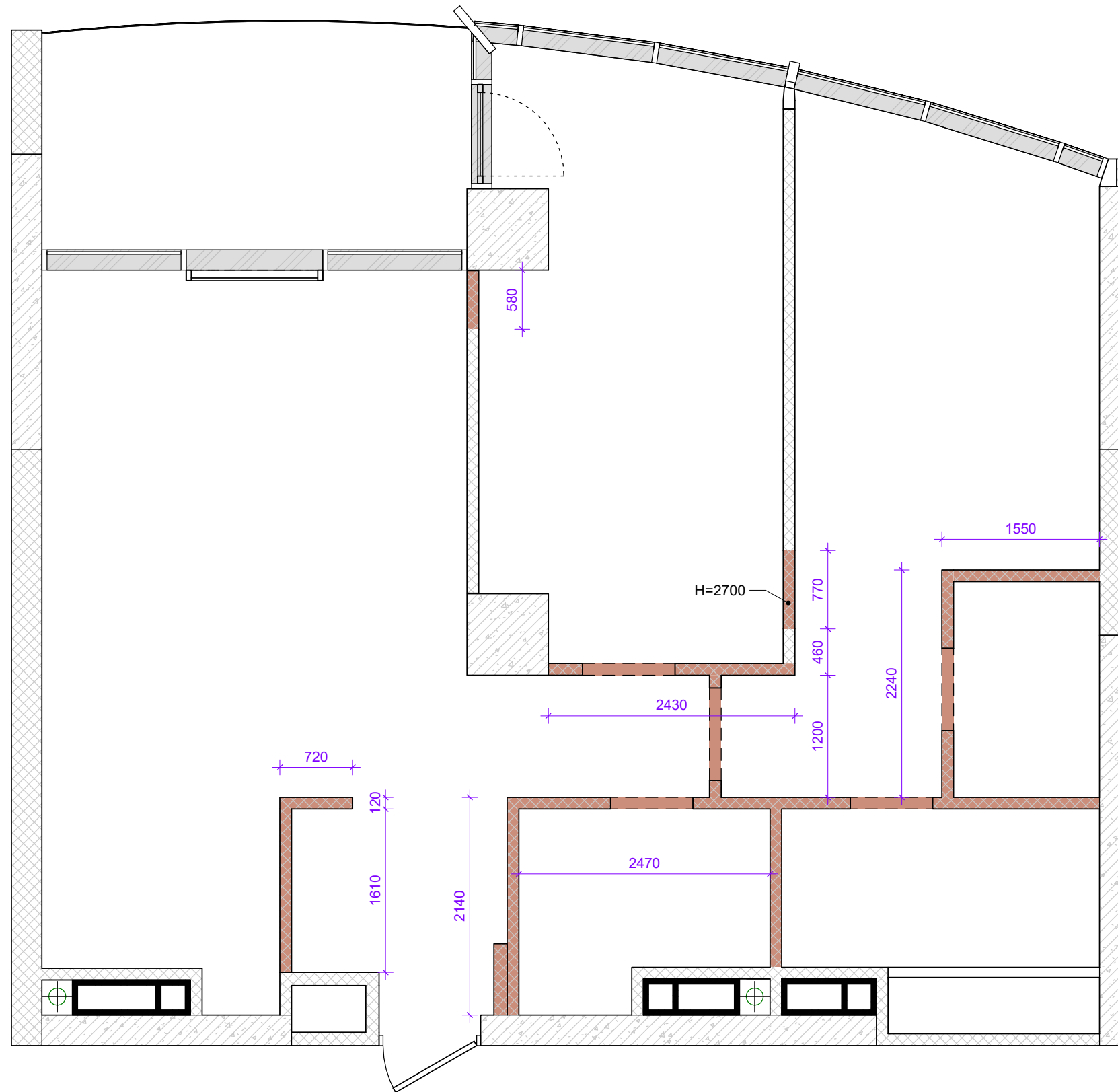
План демонтажу 1 : 50
