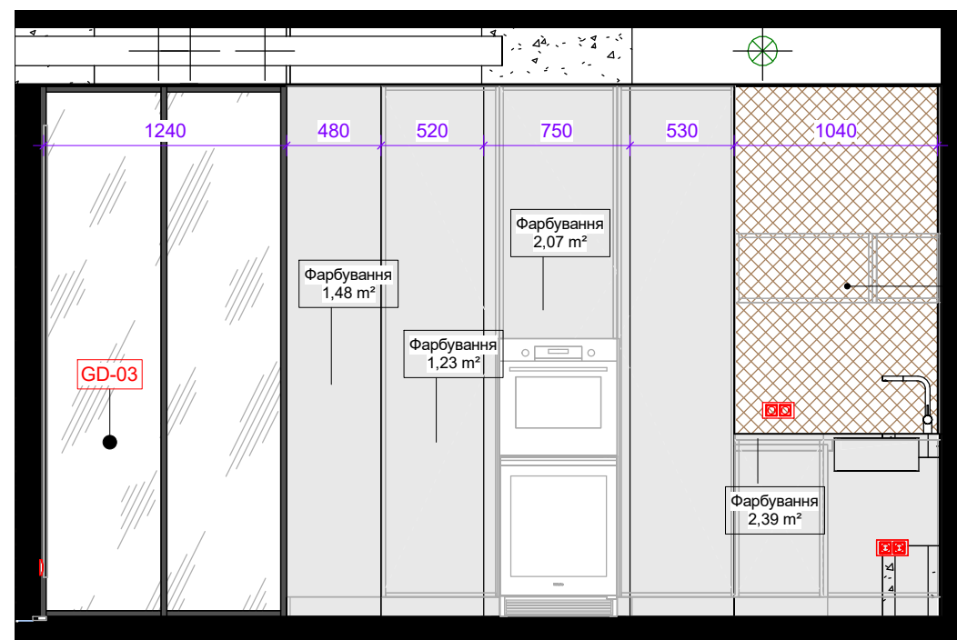
WL-02 1 : 35
