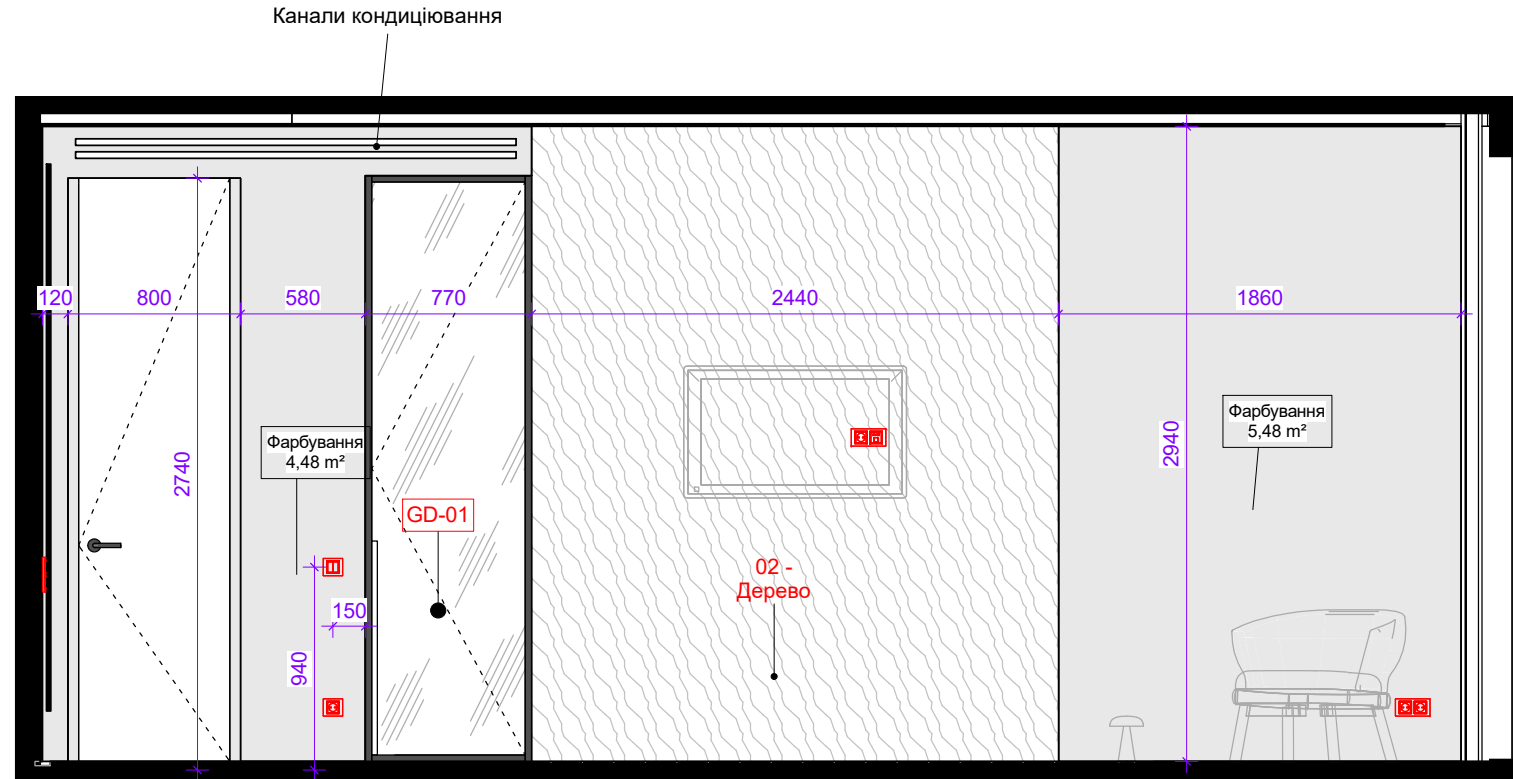
WB-02 1 : 35
