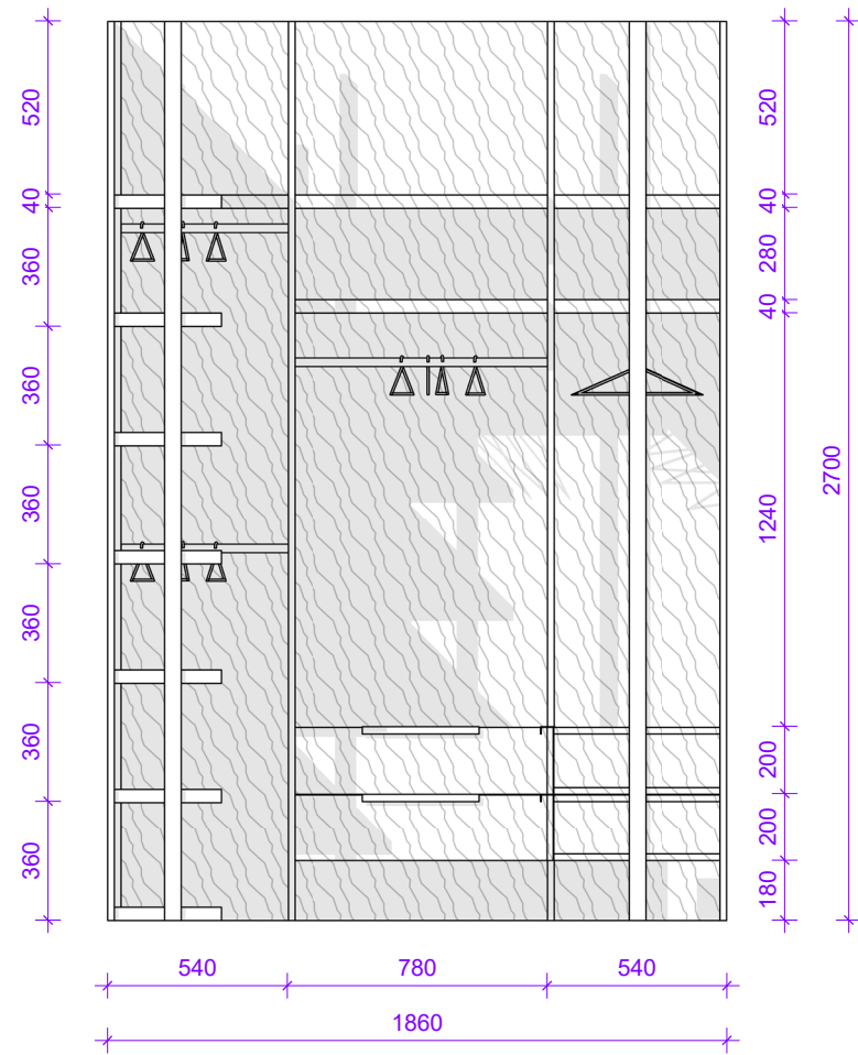
Elevation Right 1 : 25
