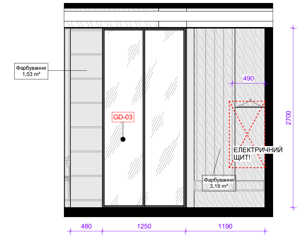
WM-08 1 : 35
