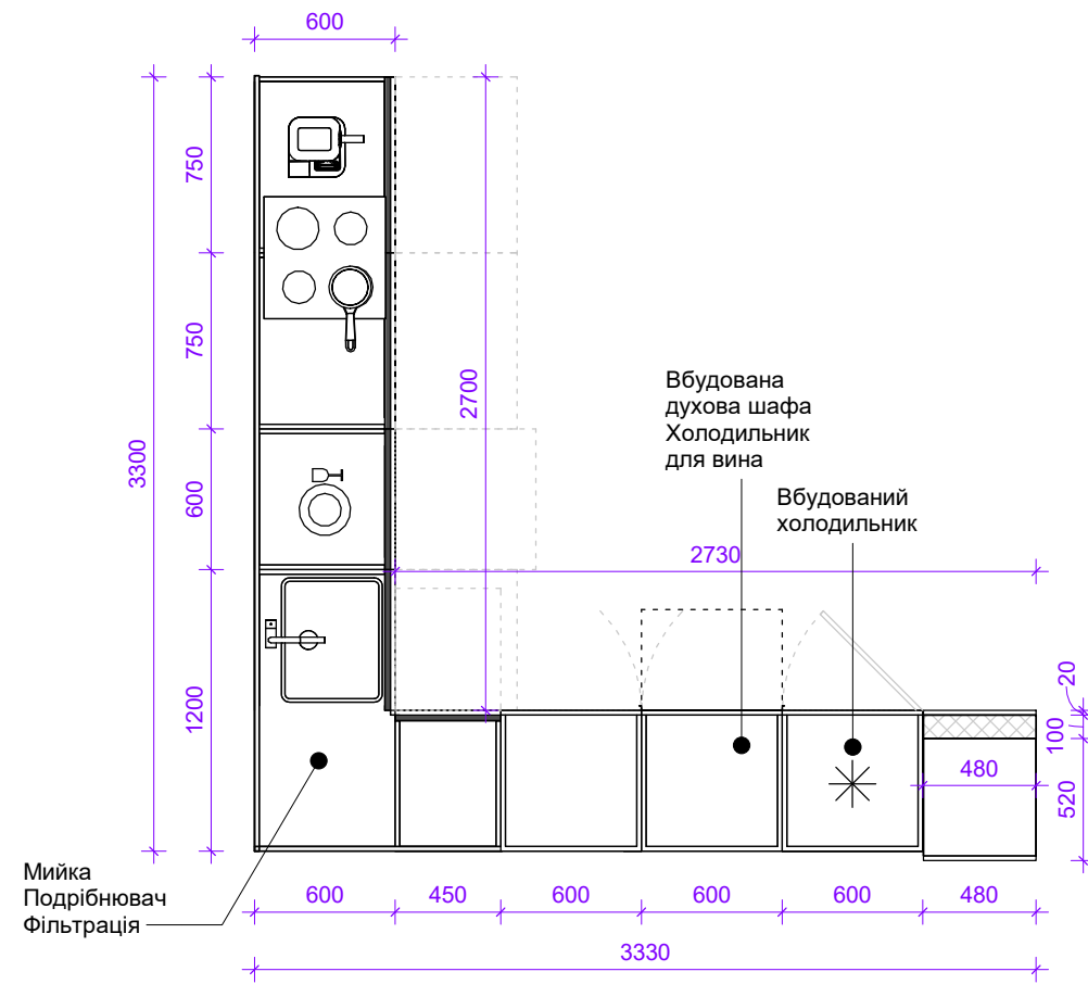
План кухні
