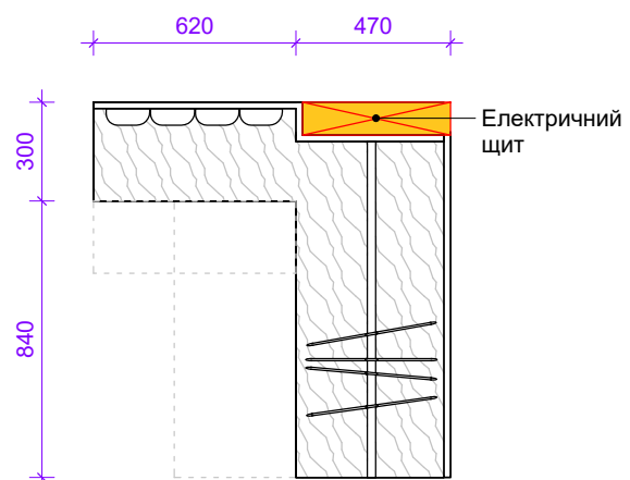
Plan Detail 1 : 25
