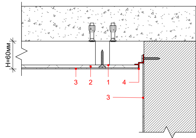
Розріз 8 (тіньовий шов)
