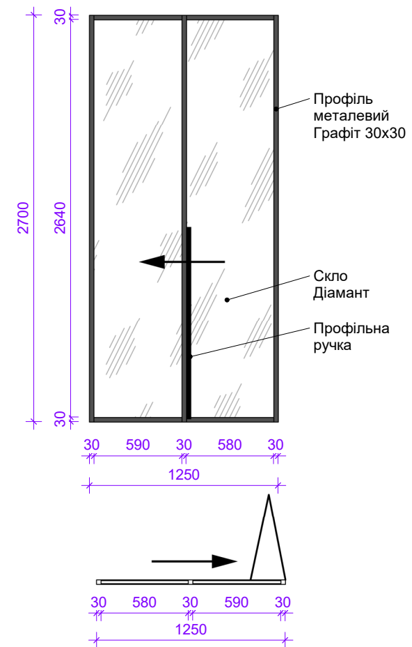
Door GD-03 M 1:35
