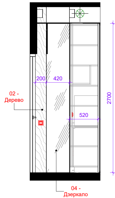
WM-07 1 : 35
