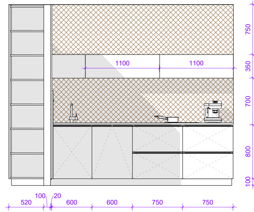
Elevation Right 1 : 35
