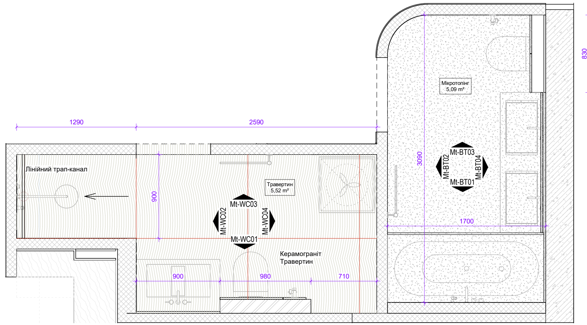
План Матеріалів Ванна й Санвузол 1 : 25
