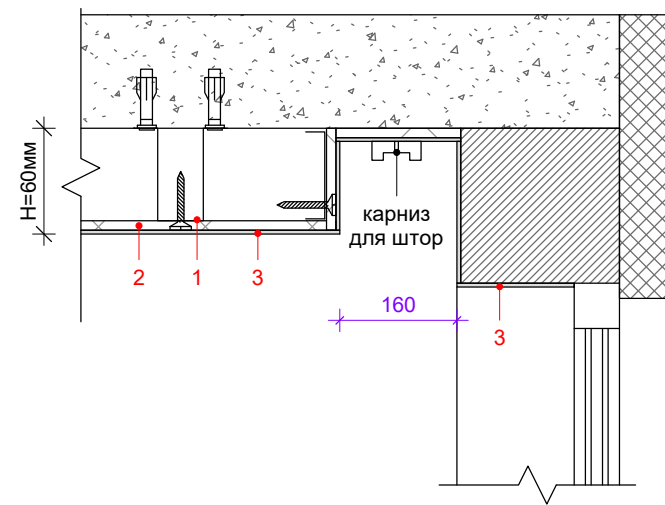
Розріз 5
