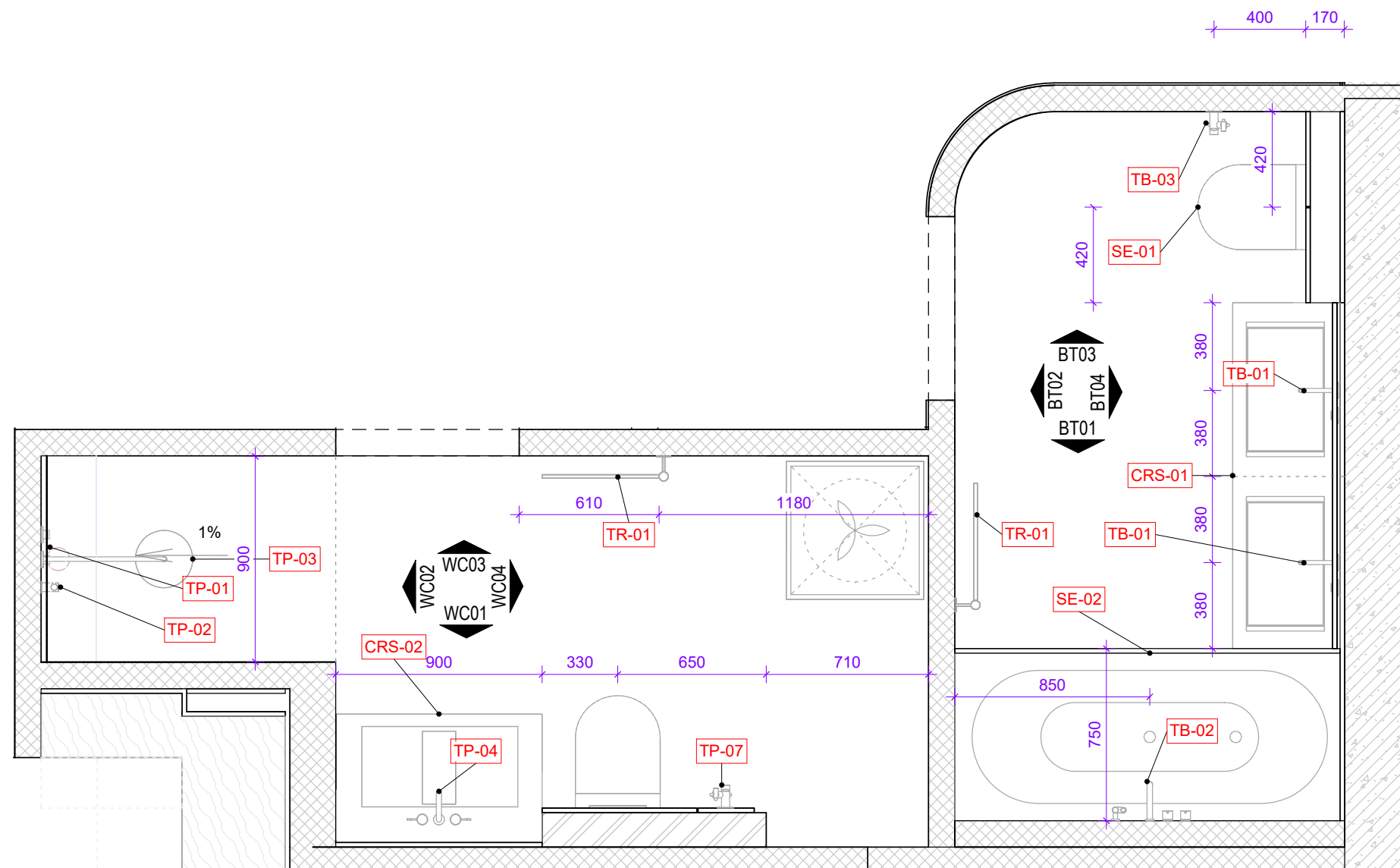
План розташування Сантехніки Ванна й Санвузол
