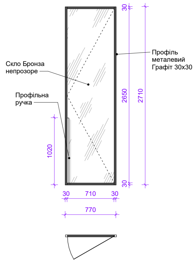
Door GD-01 M 1:35
