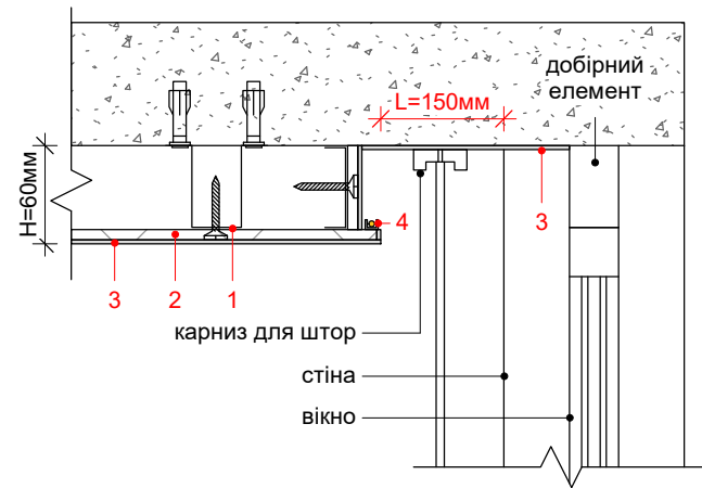
Розріз 1
