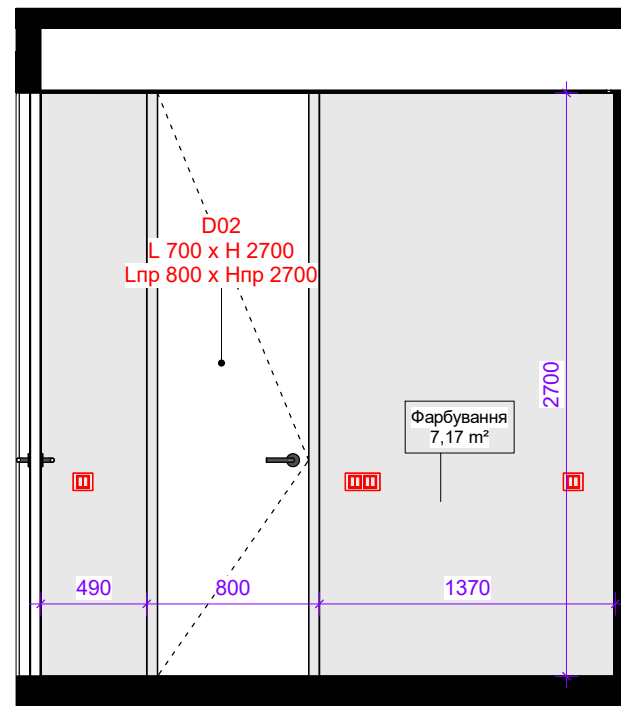
WS-01 1 : 35
