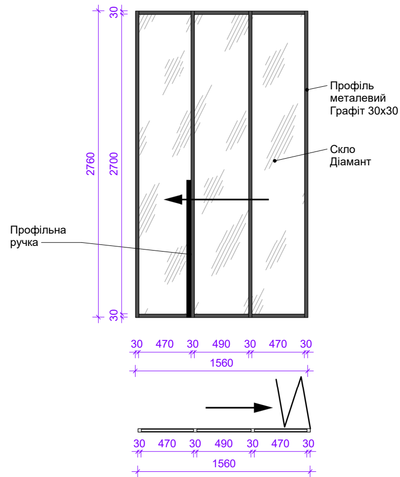
Door GD-02 M 1:35
