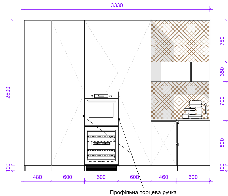
Elevation Back 1 : 35
