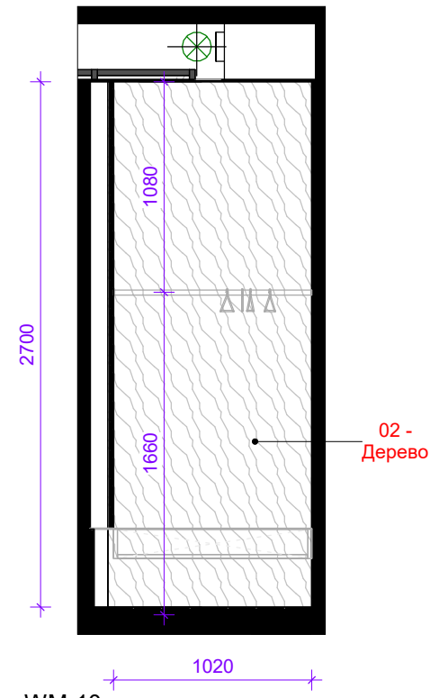
WM-10 1 : 35
