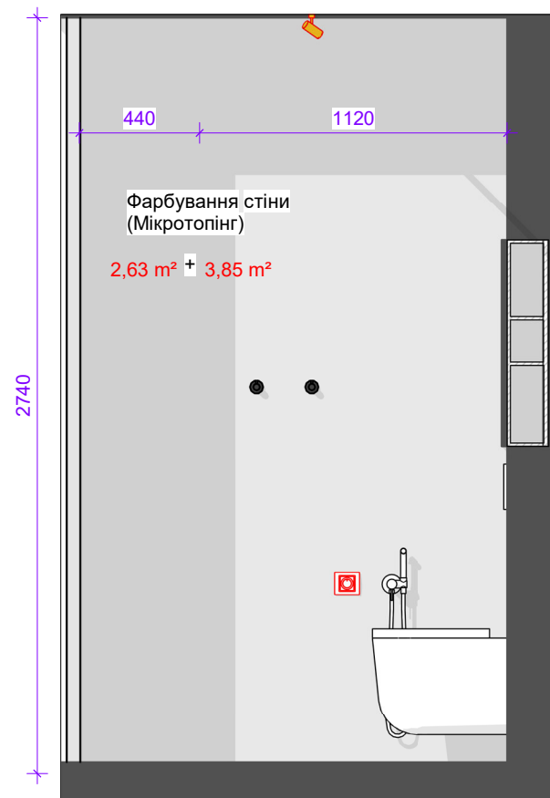
Mt-BT03 1 : 25
