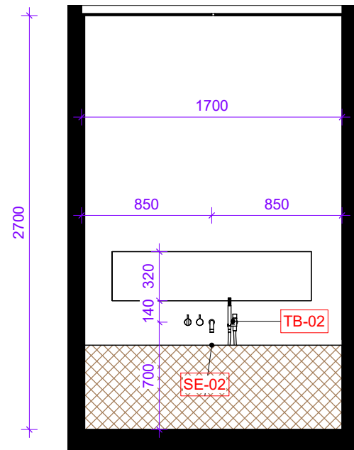
BT01 1 : 35
