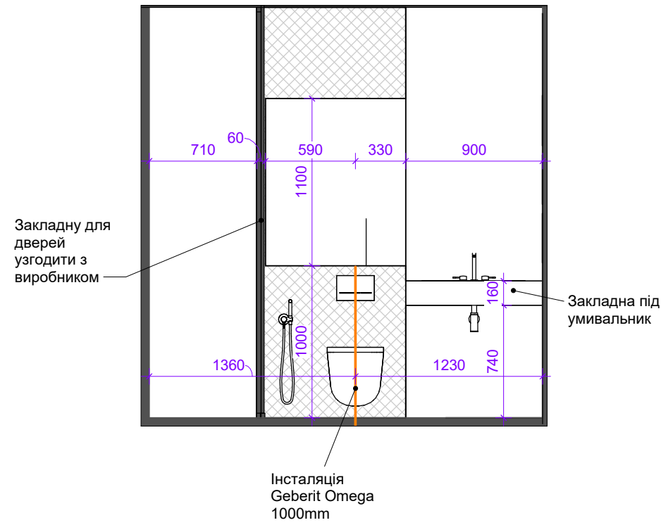
W-02 1 : 35
