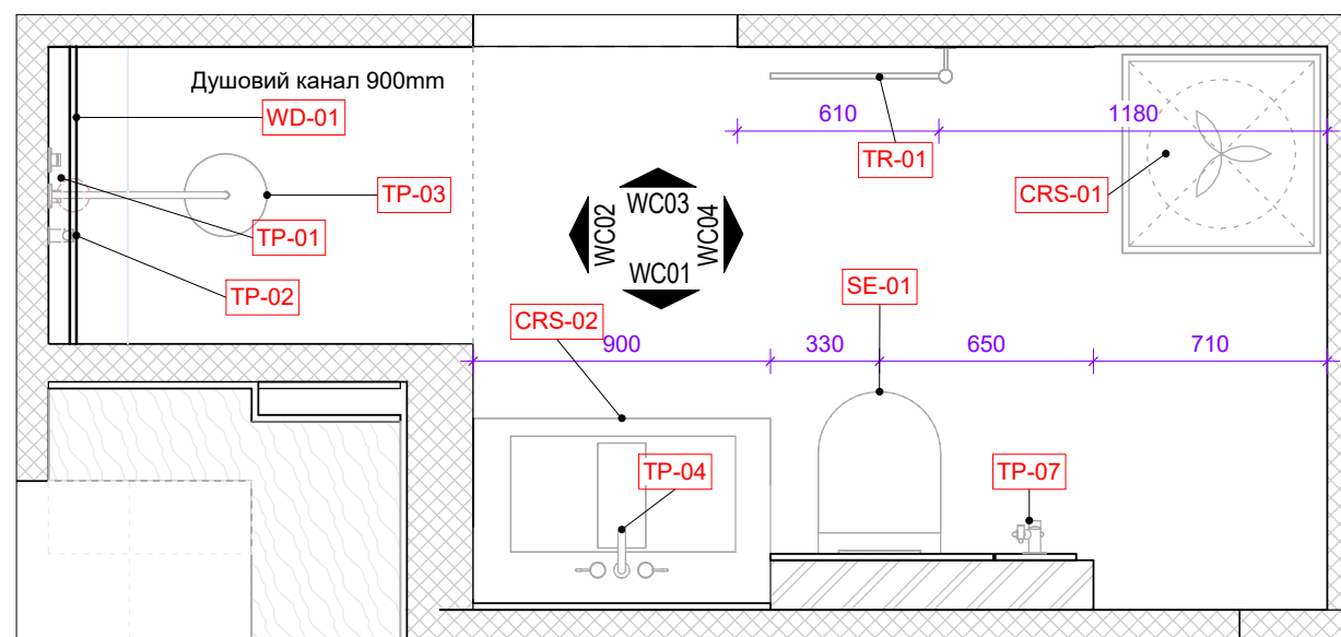
План розташування Сантехніки в Душовій 1 : 25
