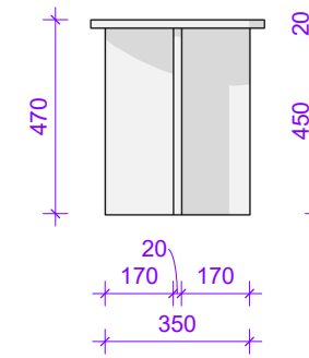
Elevation Right 1 : 20
