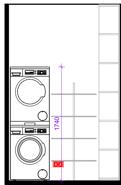
WC04 1 : 35
