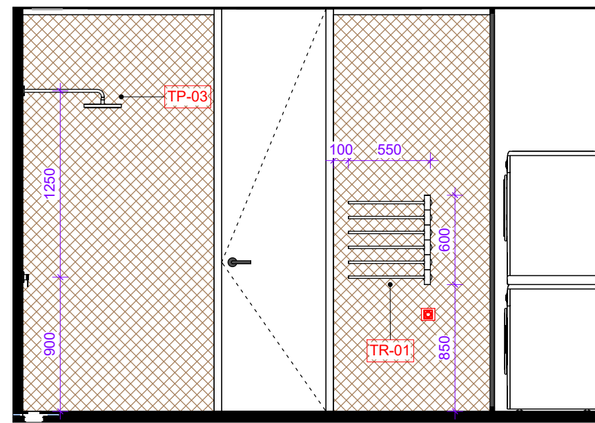
WC03 1 : 35
