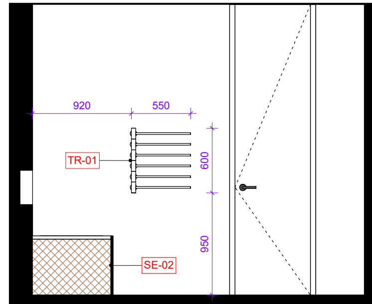
BT02 1 : 35
