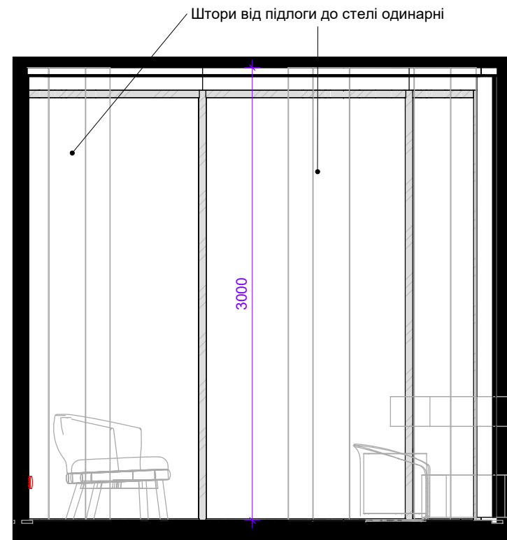
WB-03 1 : 35
