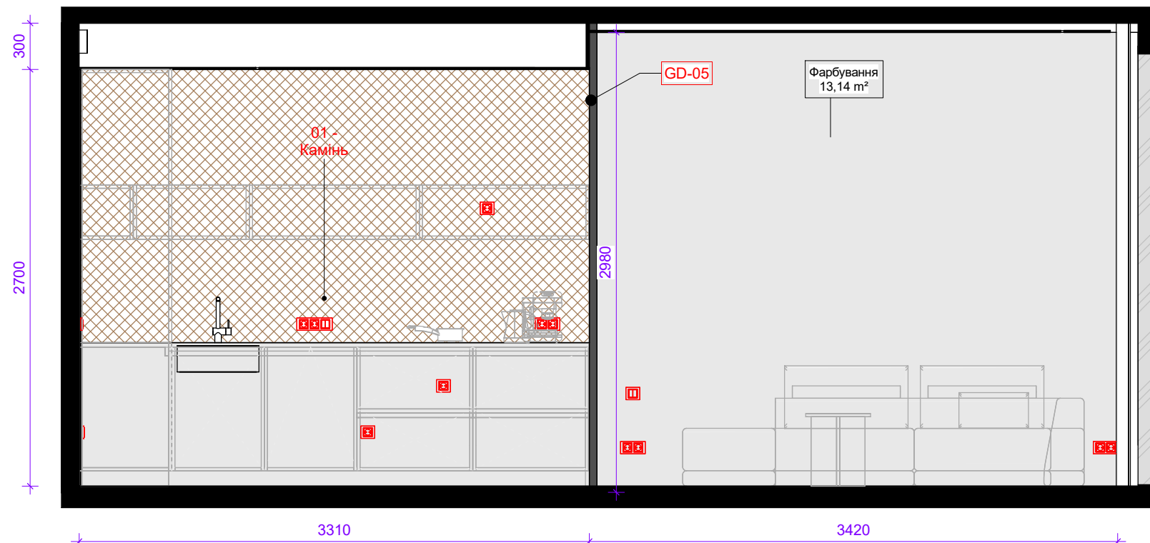
WL-01 1 : 35
