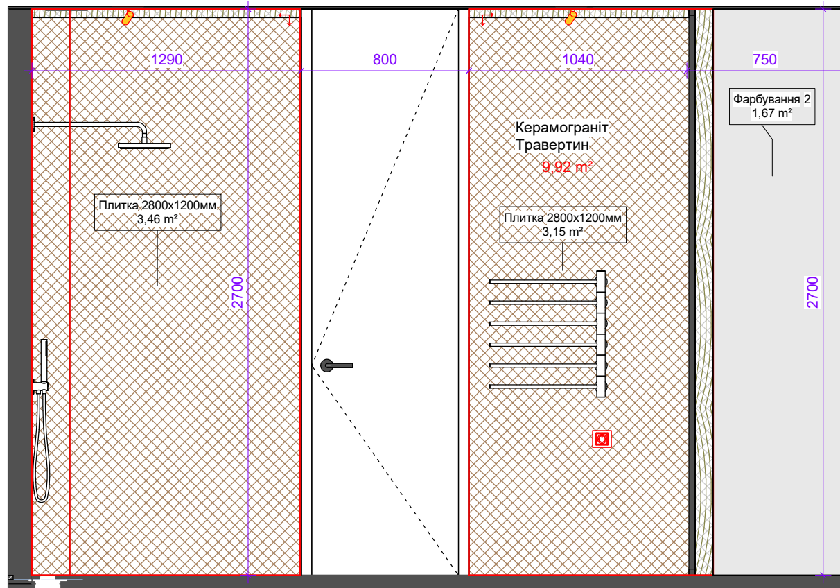
Mt-WC03
