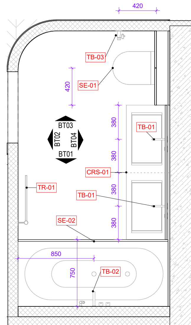
План розташування Сантехніки в Ванній 1 : 25
