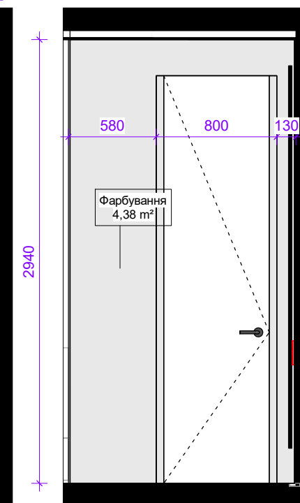
WB-05 1 : 35
