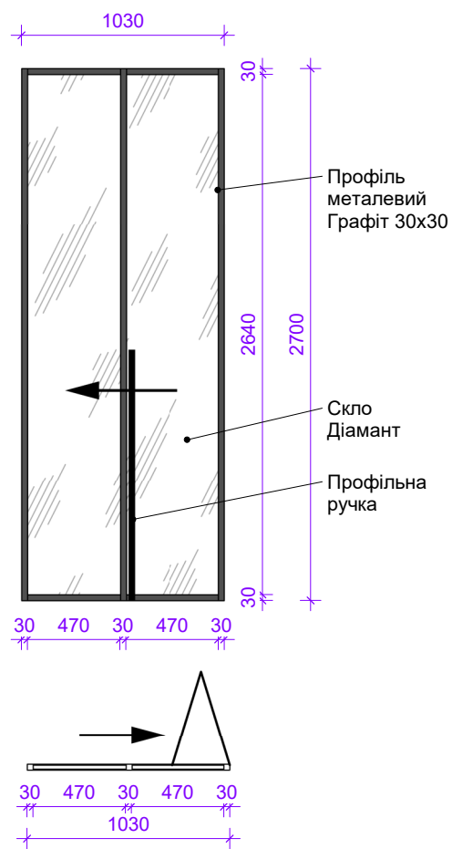
Door GD-04 M 1:35
