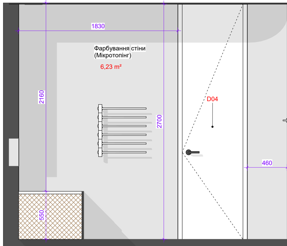
Mt-BT02 1 : 25
