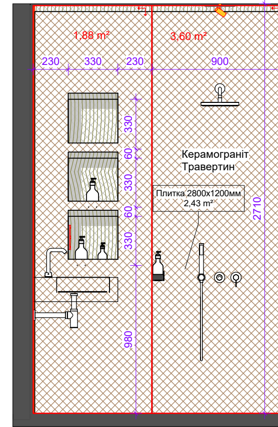
Mt-WC02
