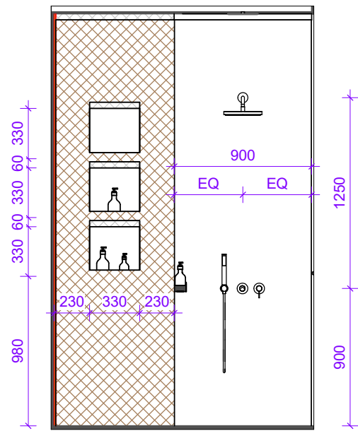
W-01 1 : 35
